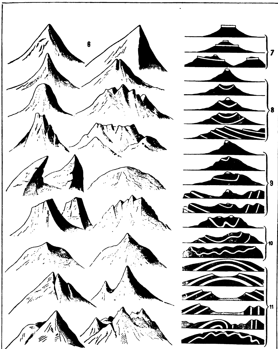
6. Typické tvary vrcholů horských (dle Sonklara v. Innstádtten). — 7.—11. Vznikání horských forem při střídajících se tvrdých (bílé) a měkkých (stínované) vrstvách dle J. P. Lesleye. — Obr. č. 7 ukazuje, jak horizontálně uložené vrstvy tvořivají v případě, že se tvrdá vrstva nalézá na povrchu, tabulové hory. Z pánvi poněkud více prohnutých vznikají dvě hory. Na obr. č. 8—10 znázorněno, jak při ostrých synklinálách tvořivá se ostrý hřbet. Je-li tvrdých vrstev více, odpovídá jim i více ostrých hřbetů. Při úplně vyvinuté pánvi shledáváme z pravidla dvakrát tolik hřbetů, co jest tvrdých vrstev. Na obr. č. 11 jeví se různé tvary vznikající při antiklinálách (sedlech).
